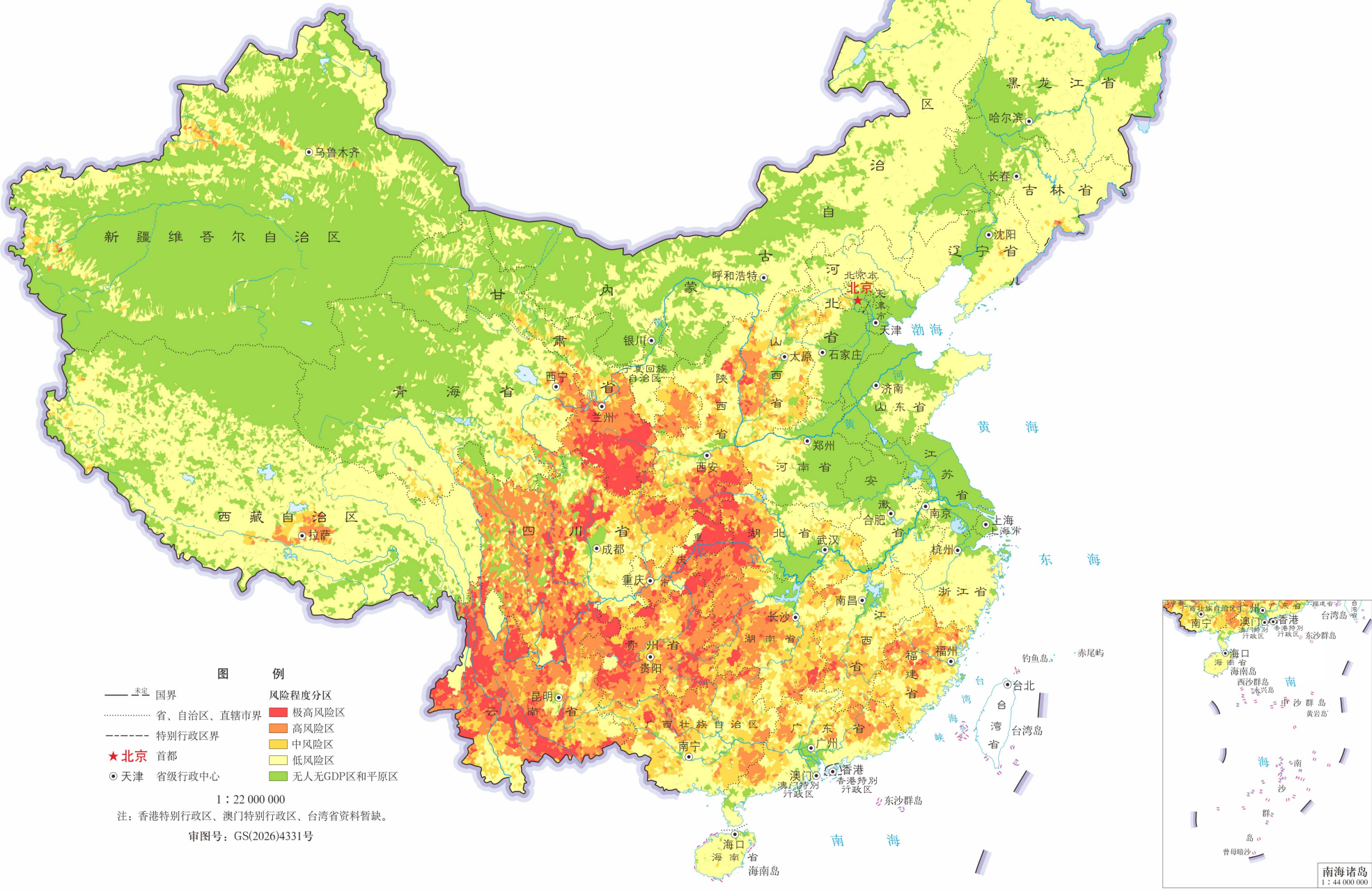
附图2 全国崩塌滑坡泥石流风险评价图
